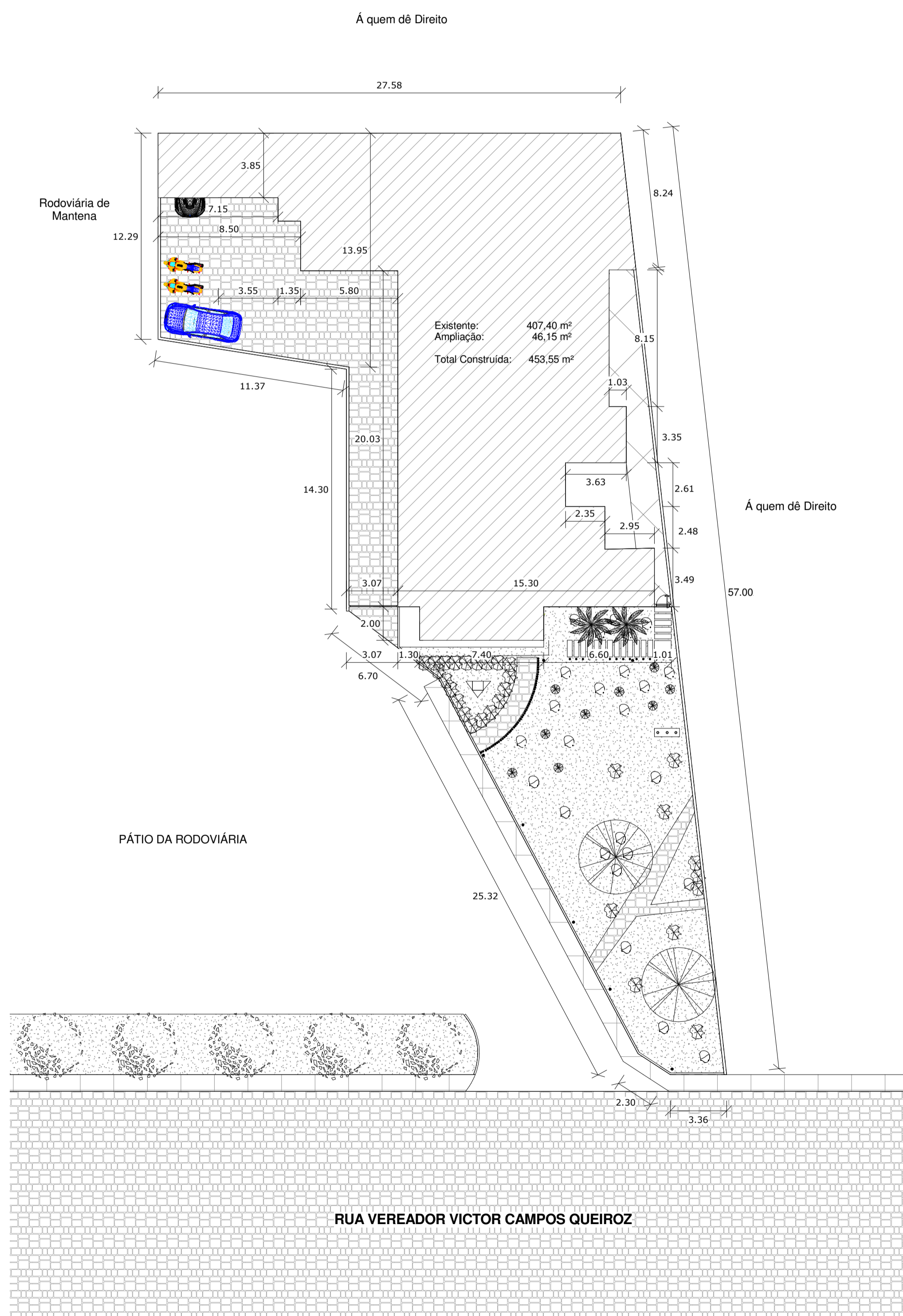
1 Planta de Situação/Implantação 1 : 200
